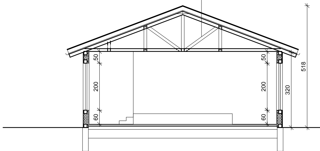
PRZEKRÓJ
